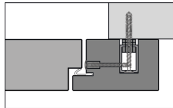
Sistema di fissaggio _ Installation System
