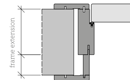
Stipite telescopico per tavolati superiori a cm 12,5 Telescopic jamb for wall thickness wider than cm 12,5
